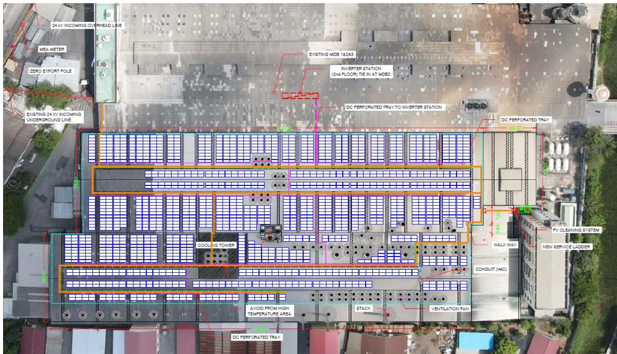
รูปที่ 1: ภาพแสดงการติดตั้งระบบผลิตไฟฟ้าจากเซลล์แสงอาทิตย์
